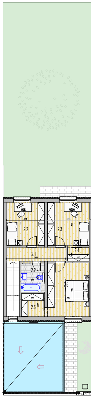
LEGENDA MIESTNOSTÍ NA 2.NP RRD TYP C2r
